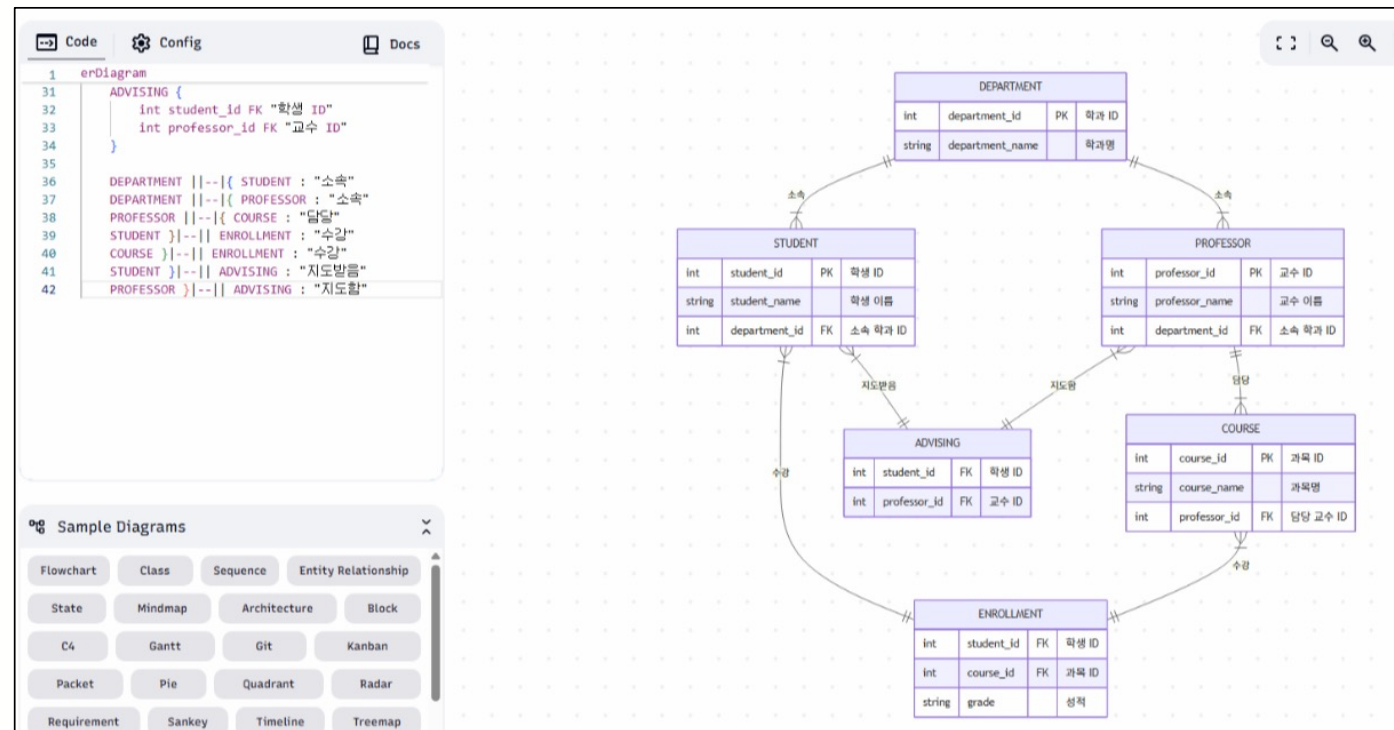
<Mermaid Chart로 그린 ER-Diagram예시>
